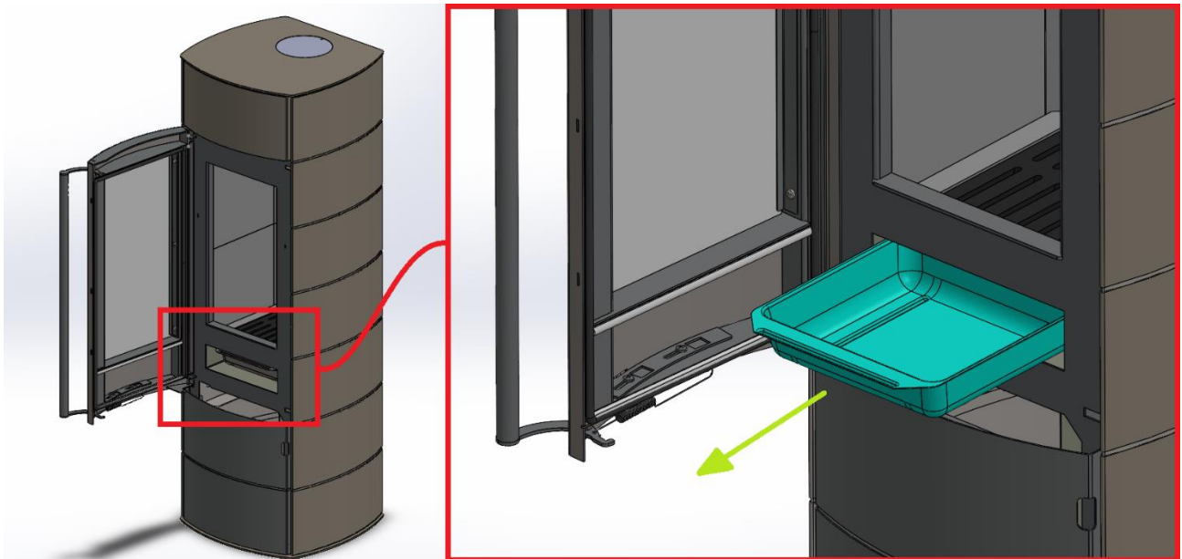
Abbildung 4 Entlären der Aschelade
